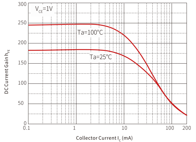
h_{FE} — I_c
