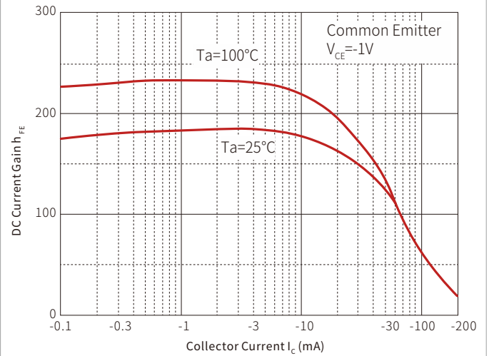
h_{FE} — I_C
